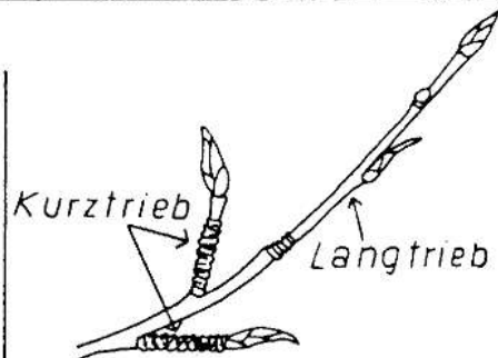
behaart
