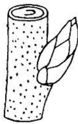
warzig (rauh)
